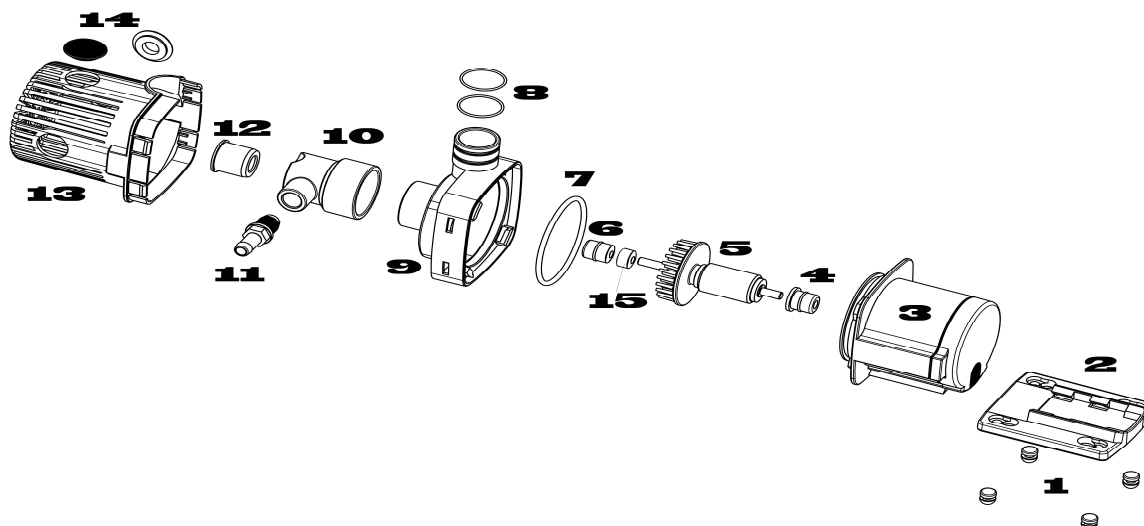
Рис. 2: Сборка насоса-диспергатора DC Runner 1.2 с 3D-крыльчаткой
