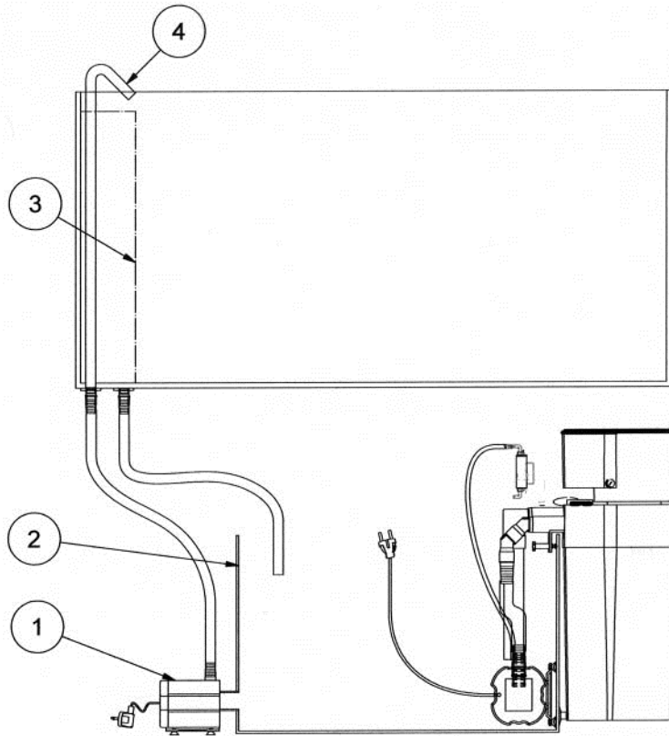
Fig. 5: EVO 1000 installatie aan de buitenzijde van de sump
