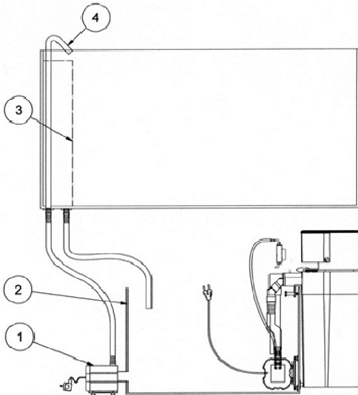
Abb. 5: EVO 1000, Aufstellung neben dem Filterbecken
