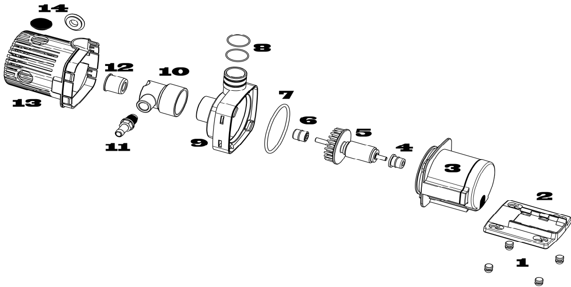
Fig. 2: Venturi pomp DC Runner 1.2 incl. 3D-naald wiel
