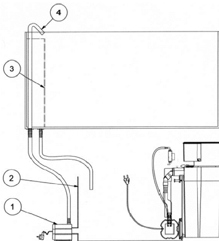
Рис. 5: EVO 1000, установка рядом с фильтрационной камерой
