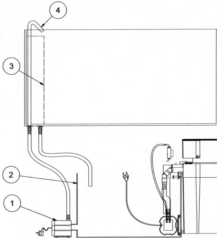
Fig. 5: Instalación de EVO 1000 en tanque de filtración
