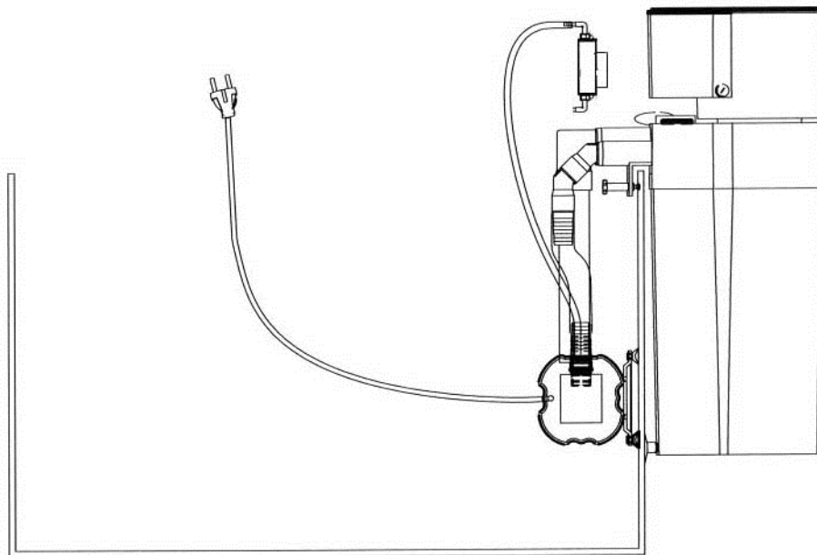
Schéma 4: EVO 1000 accroché comme écumeur extérieur
