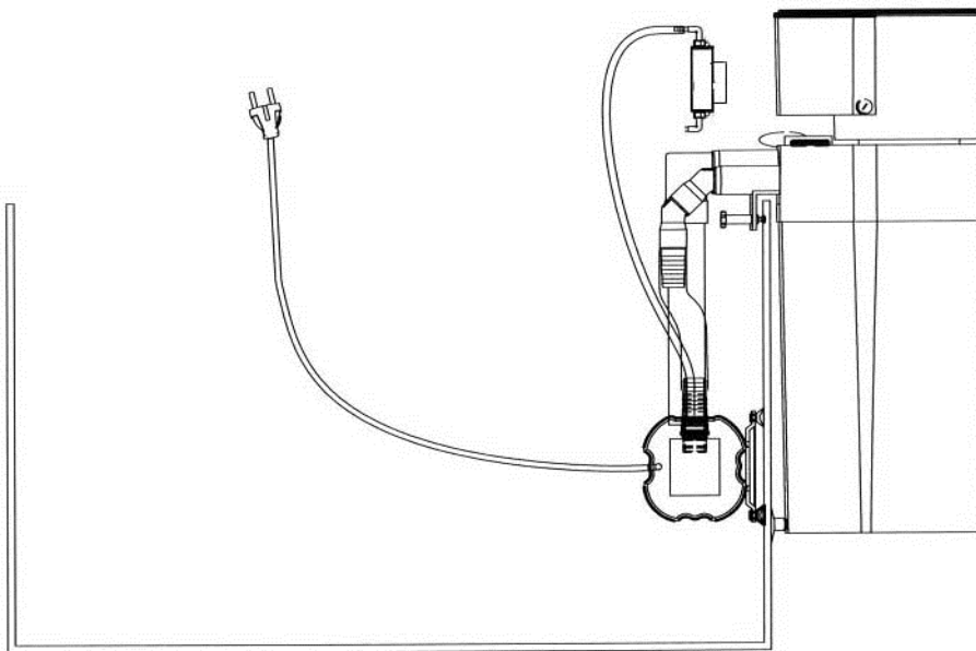
Рис. 4: EVO 1000 навесной, внешний флотатор
