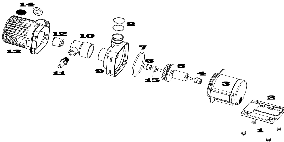
Abb. 2: Aufbau der Dispergatorpumpe DC Runner 1.2 mit 3D-Nadelrad
