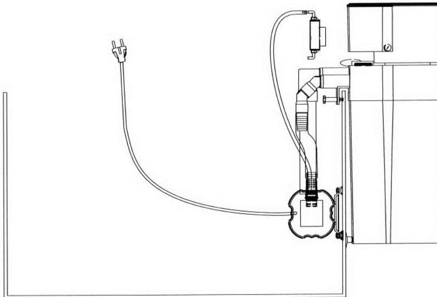
Fig. 4: EVO 1000 en operación "Colgado"
