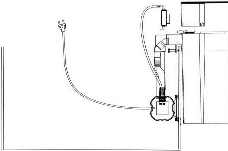
Abb. 4: EVO 1000 als Außenabschäumer, angehängt
